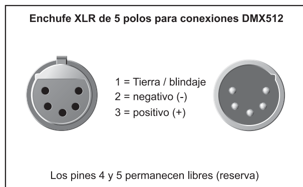
Fig. 4.1: Asignación de pins en un conector XLR de 5 polos
